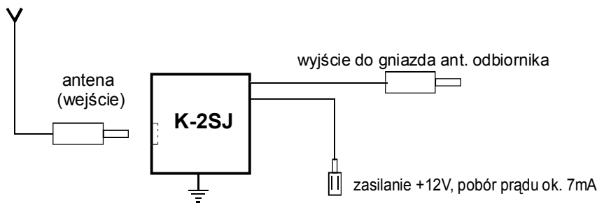
Schemat podłączenia konwertera
